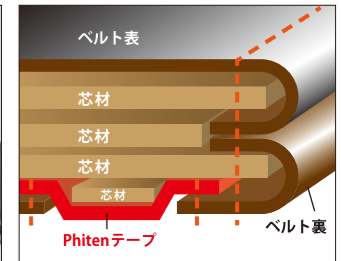
ベルト表 芯材 芯材 芯材 芯材 Phitenテープ ベルト裏
